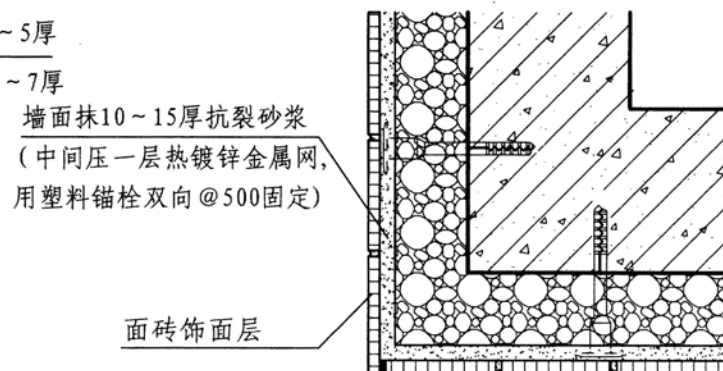
3 阳角（面砖）
