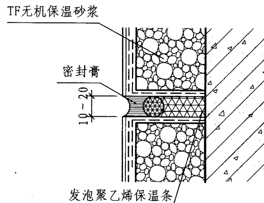
1 系统变形缝
