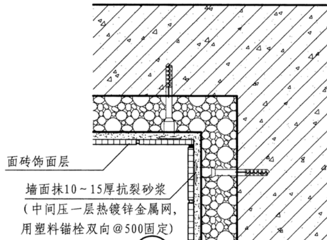
4 阴角（面砖）
