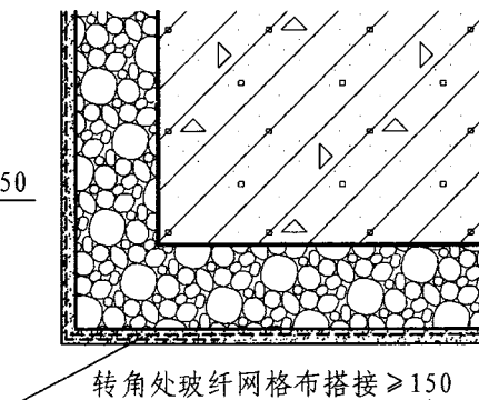
② 阳角
