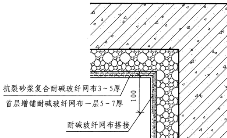
2 阴角（涂料）
