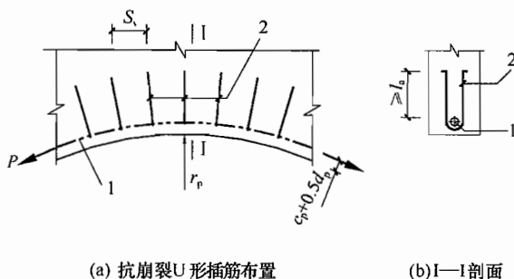
图 10.3.11 抗崩裂 U 形插筋构造示意
