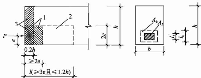
图 10.3.8 防止端部裂缝的配筋范围
