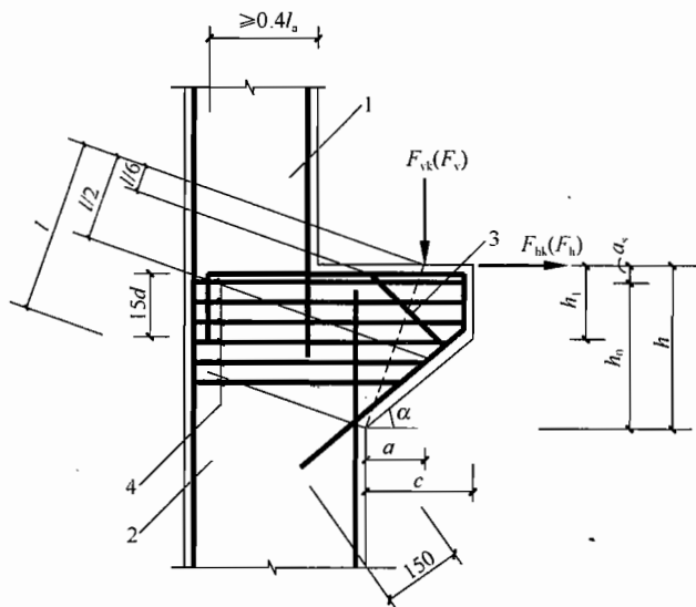
图 9.3.10 牛腿的外形及钢筋配置
