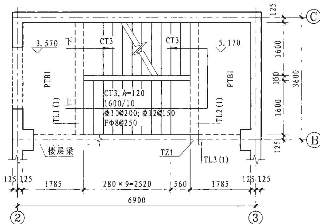
图2 设计示例 \nabla 3.570 - \nabla 5.170 楼梯平面图
