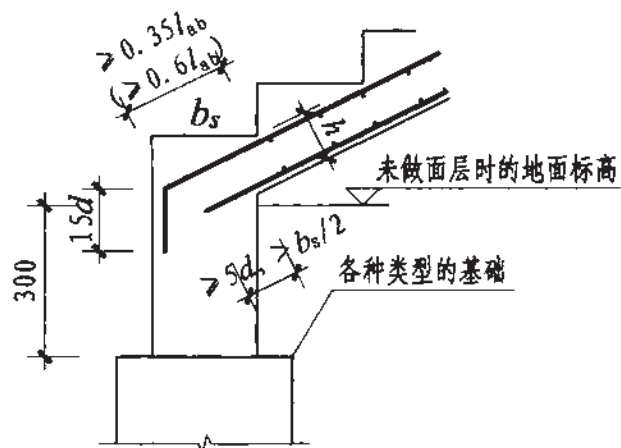
各型楼梯第一跑与基础连接构造一
