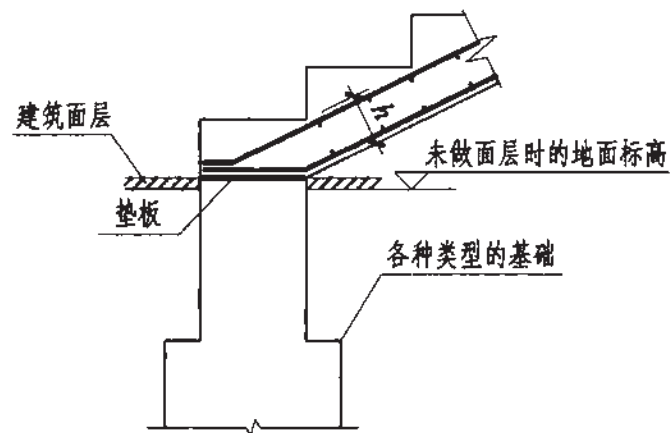
各型楼梯第一跑与基础连接构造三
