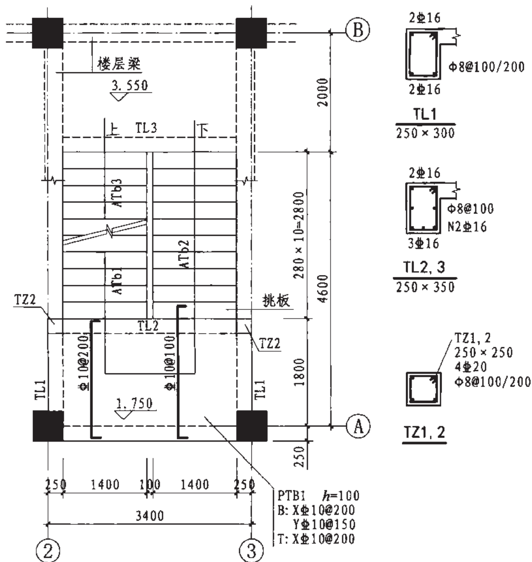
二层平面图
