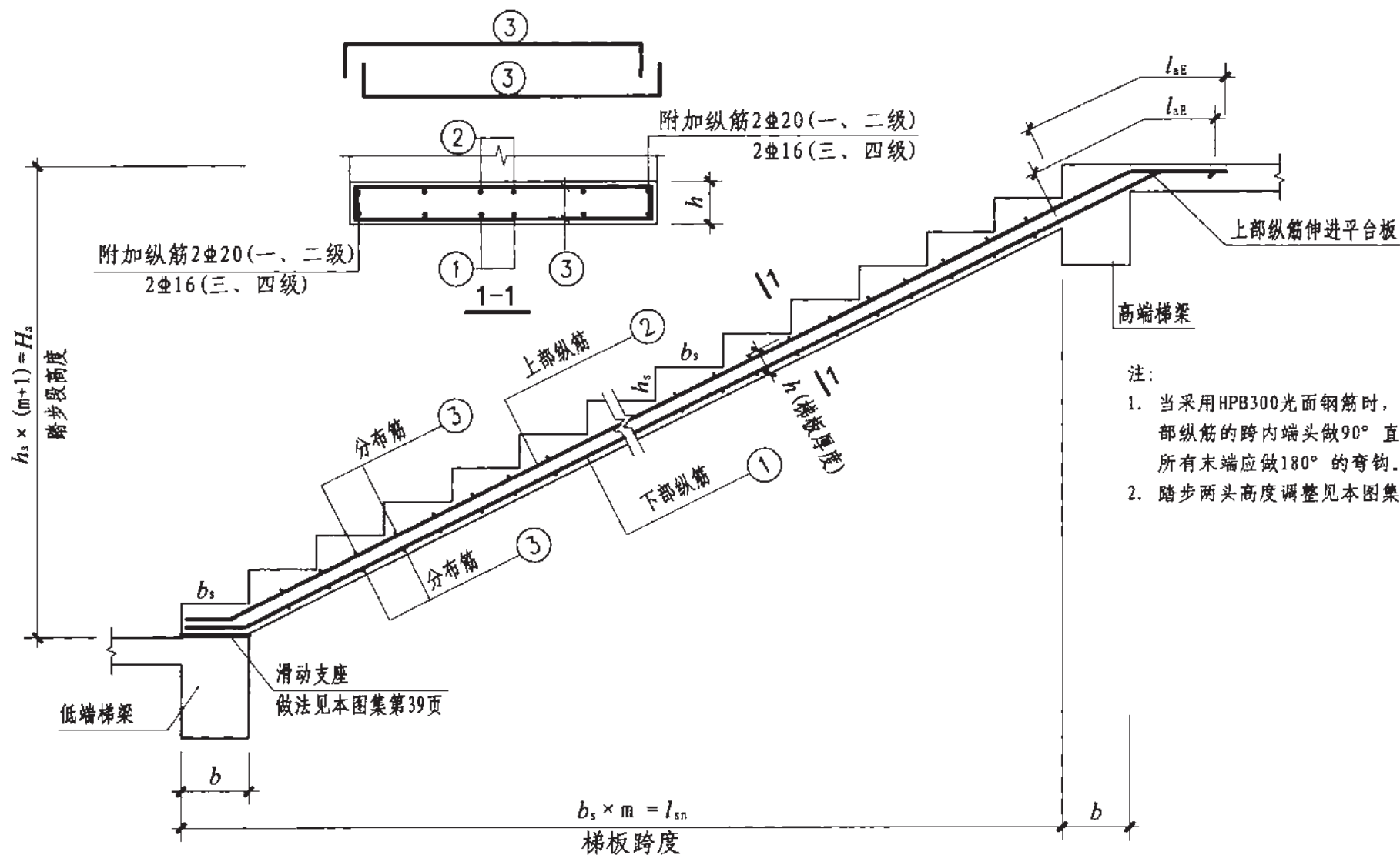
ATa楼梯板配筋构造
