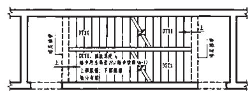
图4 交叉楼梯(无层间平台板)
