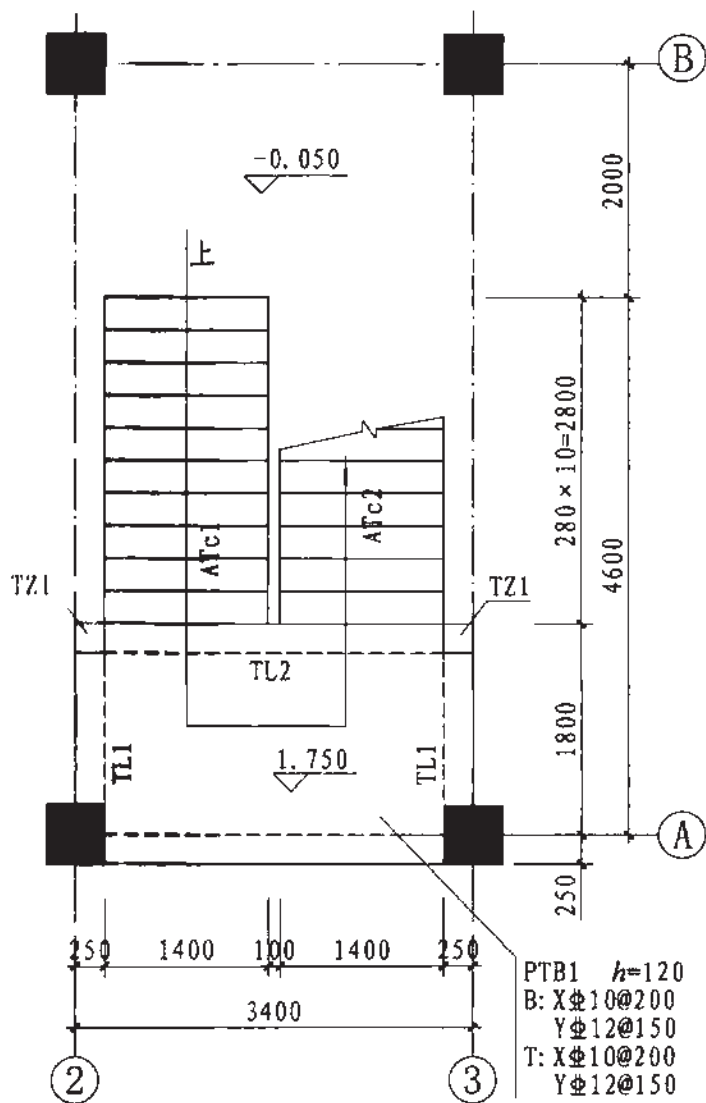
一层平面图
