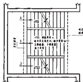
图3 双分平行楼梯
