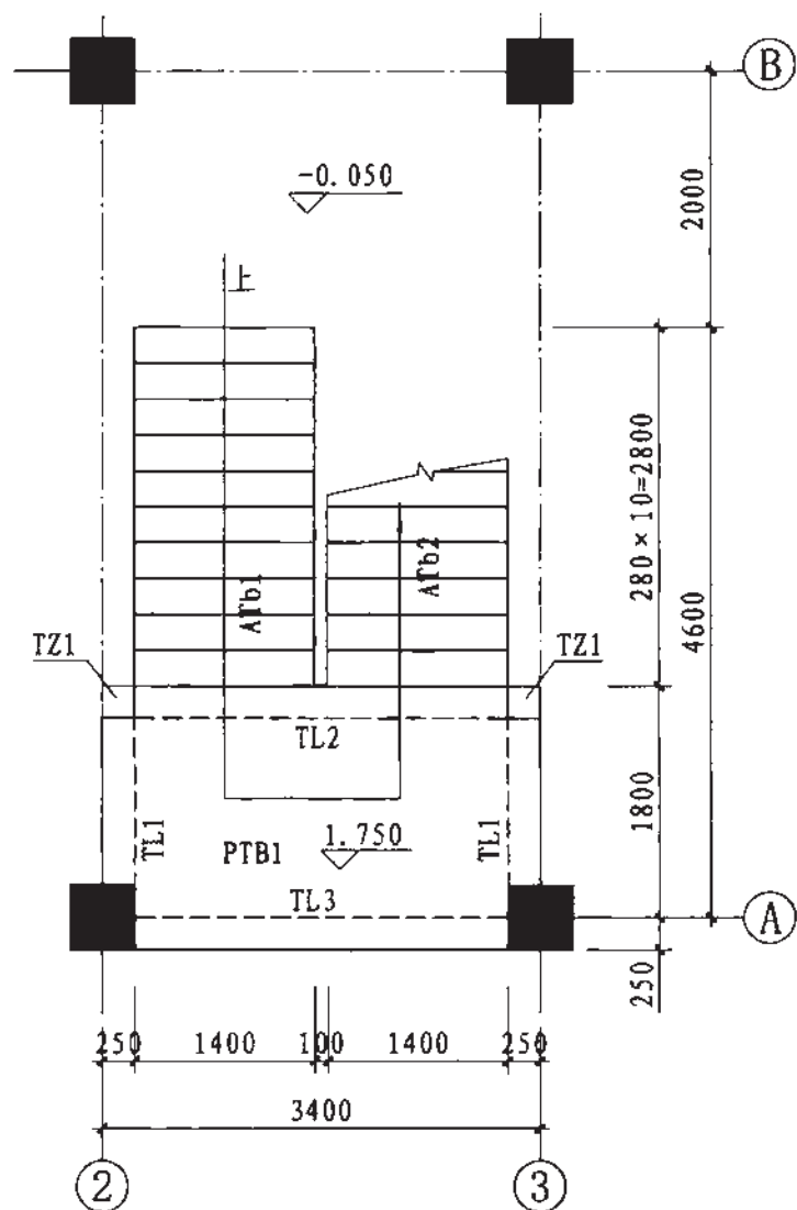
一层平面图
