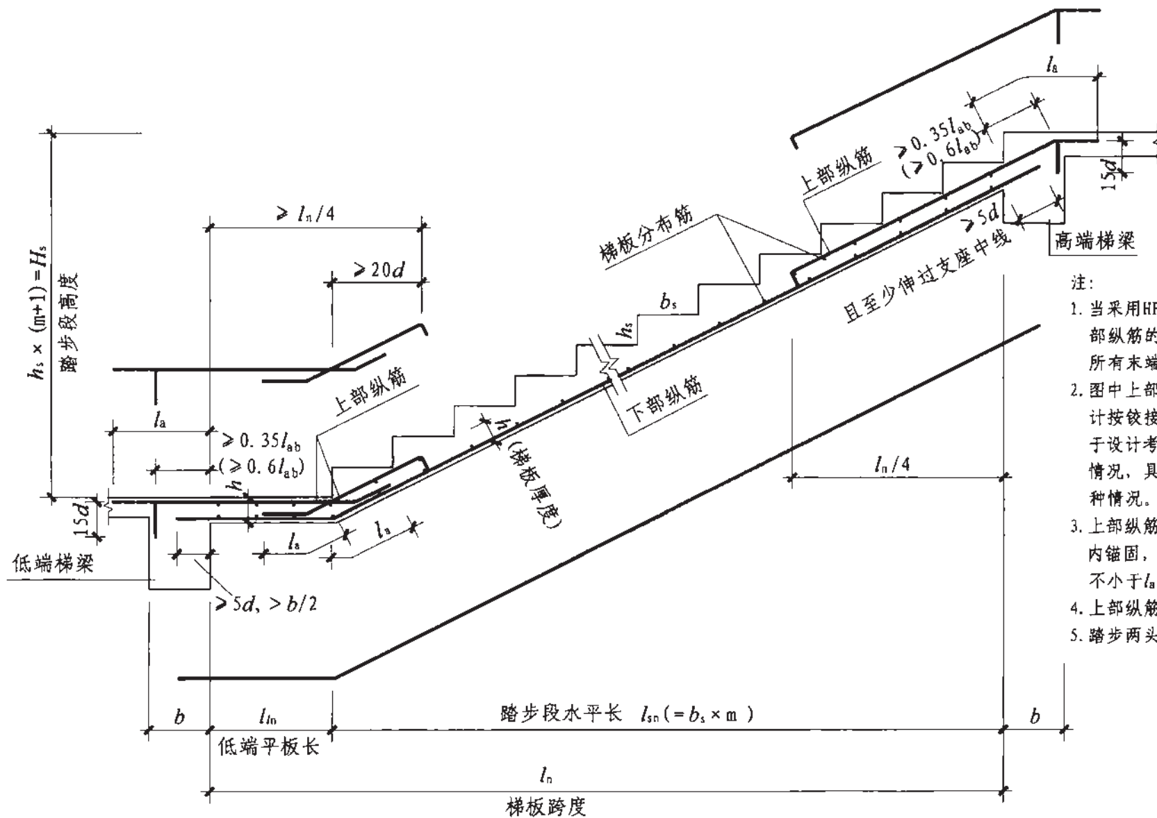
BT型楼梯板配筋构造
