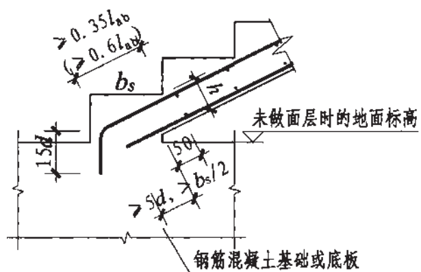
各型楼梯第一跑与基础连接构造二
