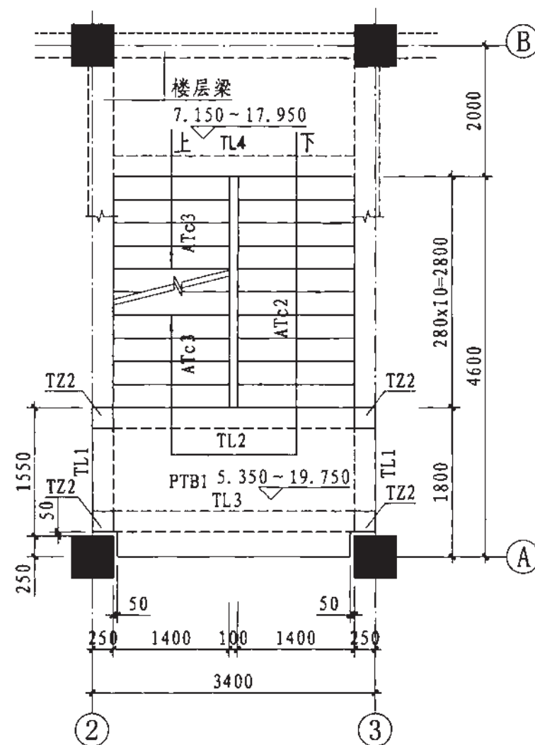
标准层平面图
