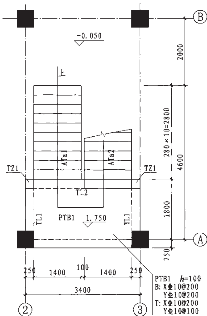
一层平面图
