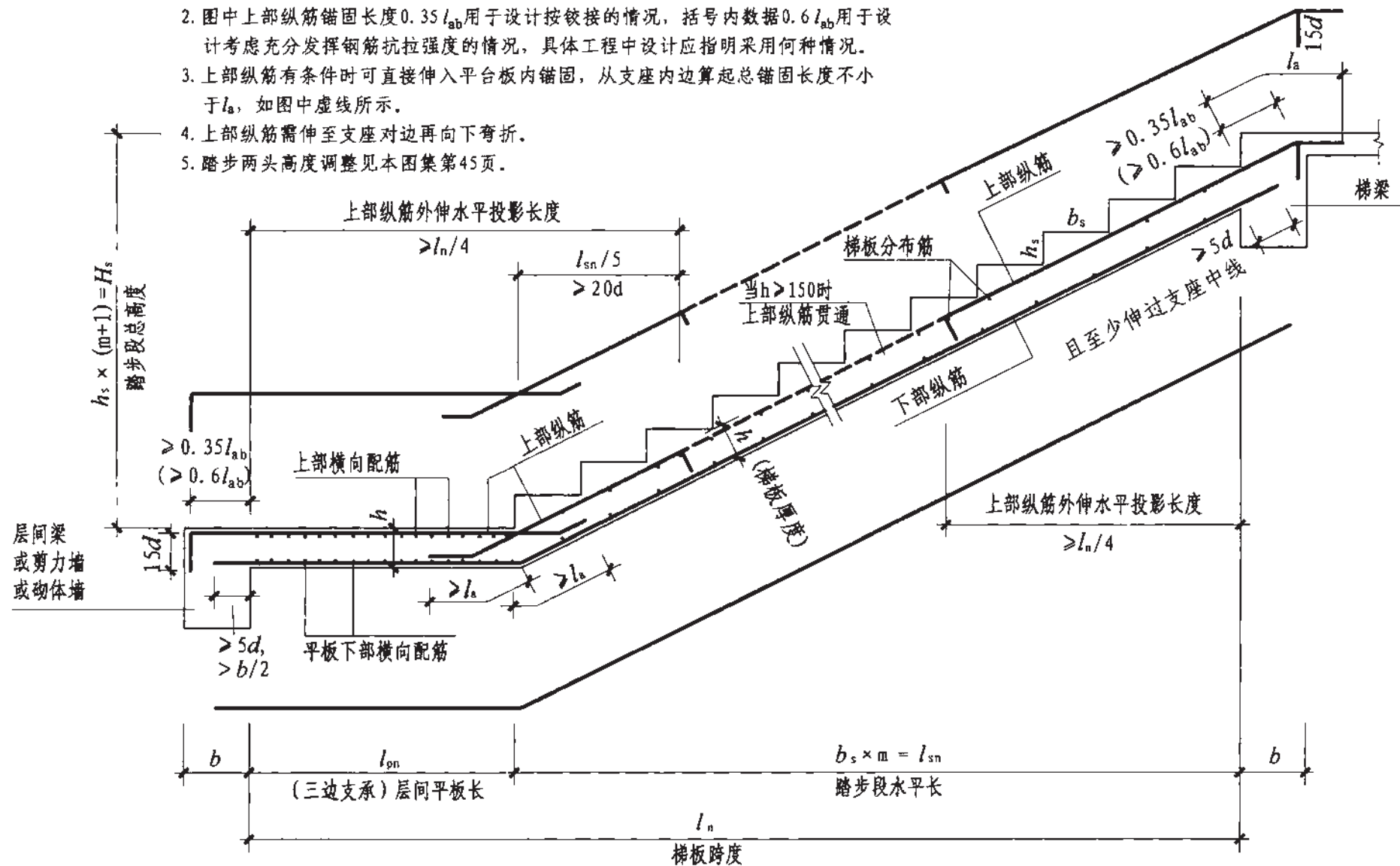
HT型楼梯板配筋构造(B-B) (层间平板为三边支承，踏步段楼层端为单边支承)
