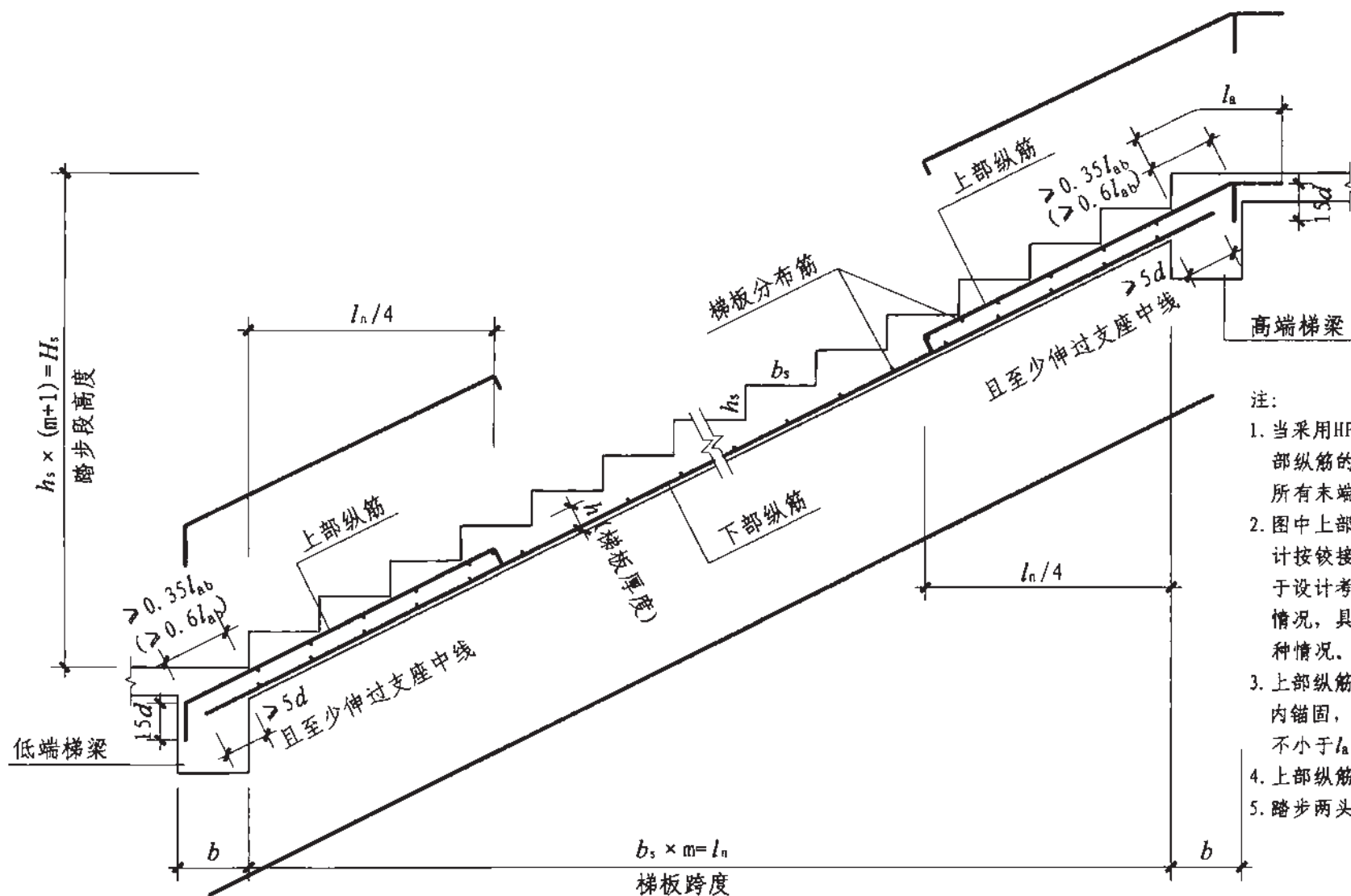
AT型楼梯板配筋构造
