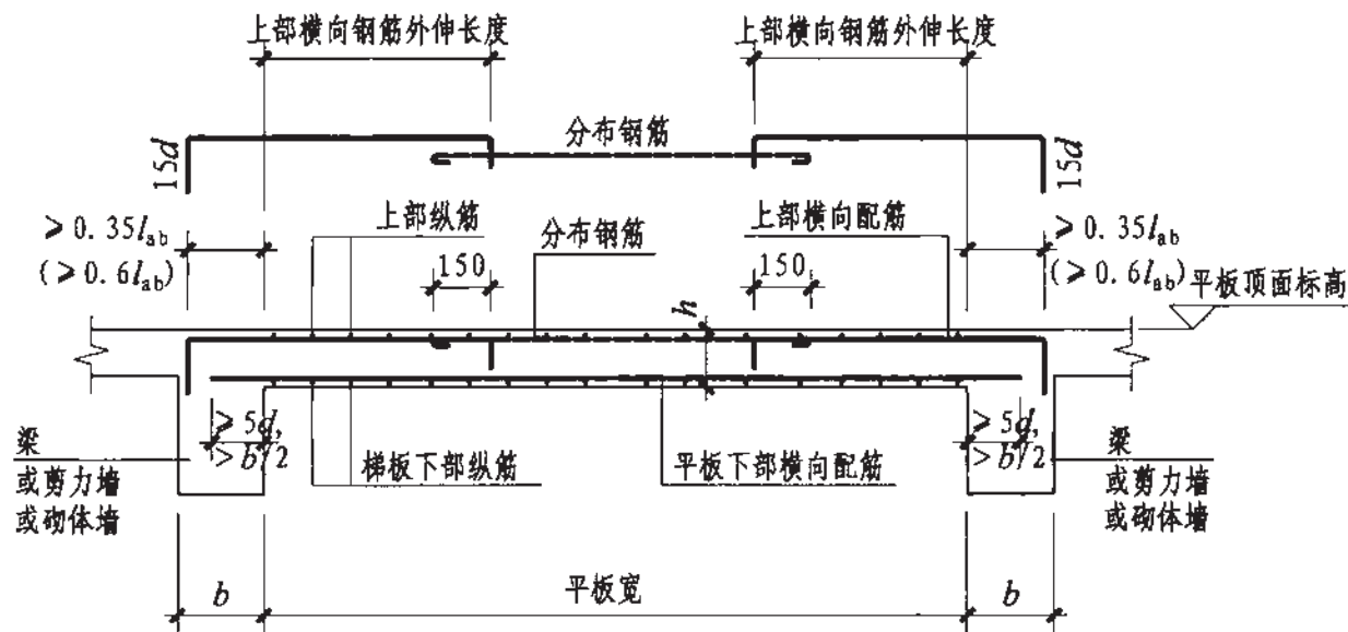
C-C剖面楼梯平板配筋构造
