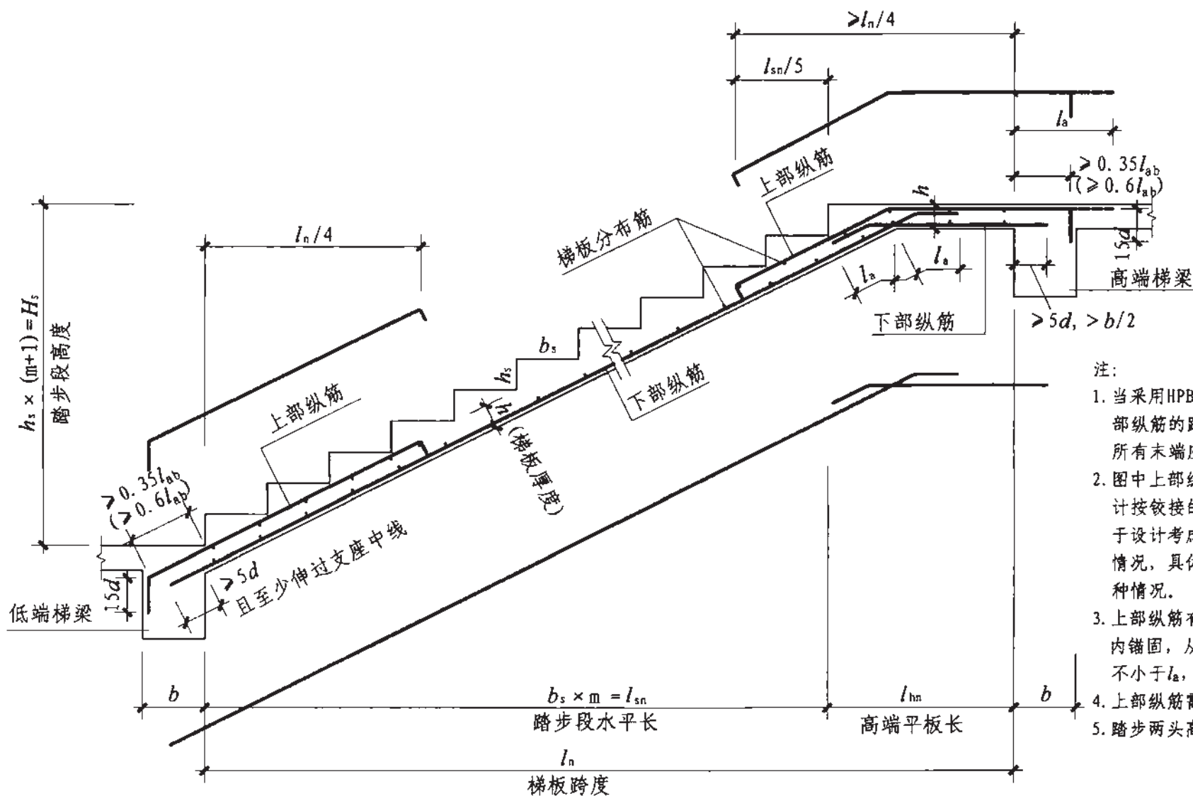
CT型楼梯板配筋构造
