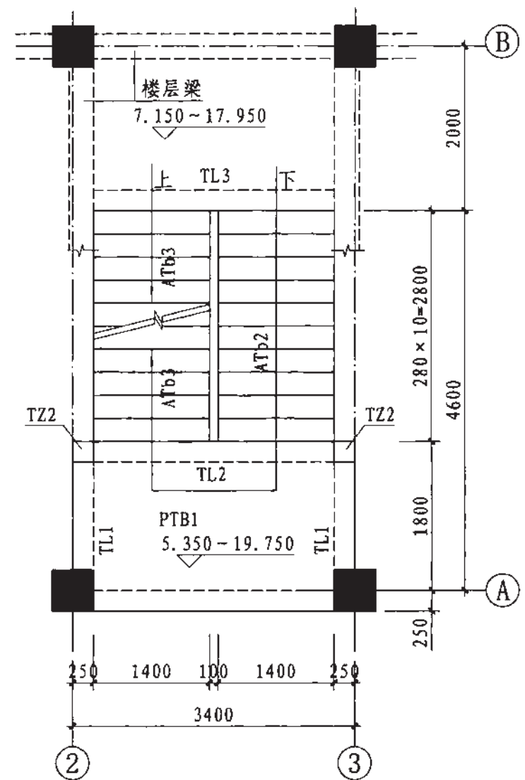
标准层平面图
