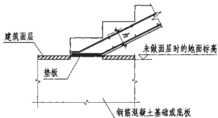
各型楼梯第一跑与基础连接构造四
