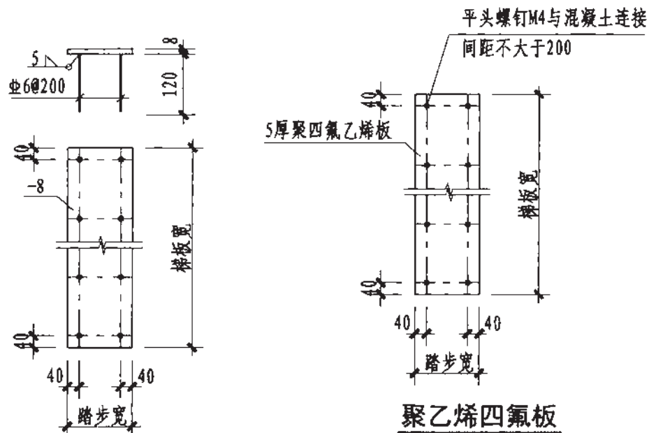
(2) 设聚四氟乙烯垫板 (梯段浇筑时应在垫板上铺塑料薄膜)
