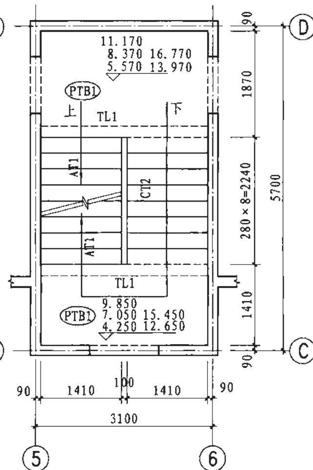
标准层楼梯平面图
