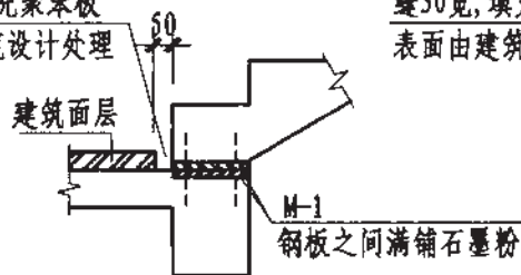
(1) 预埋钢板
