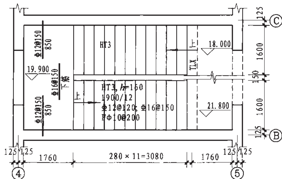
图2 设计示例 标高18.000—标高21.800楼梯平面图
