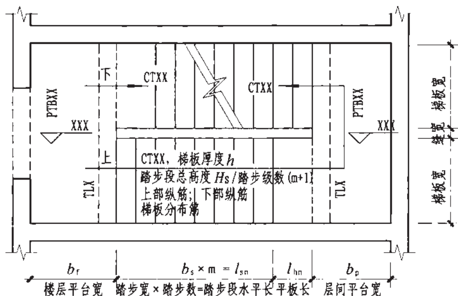
图1 注写方式 ▽XXX—▽XXX楼梯平面图
