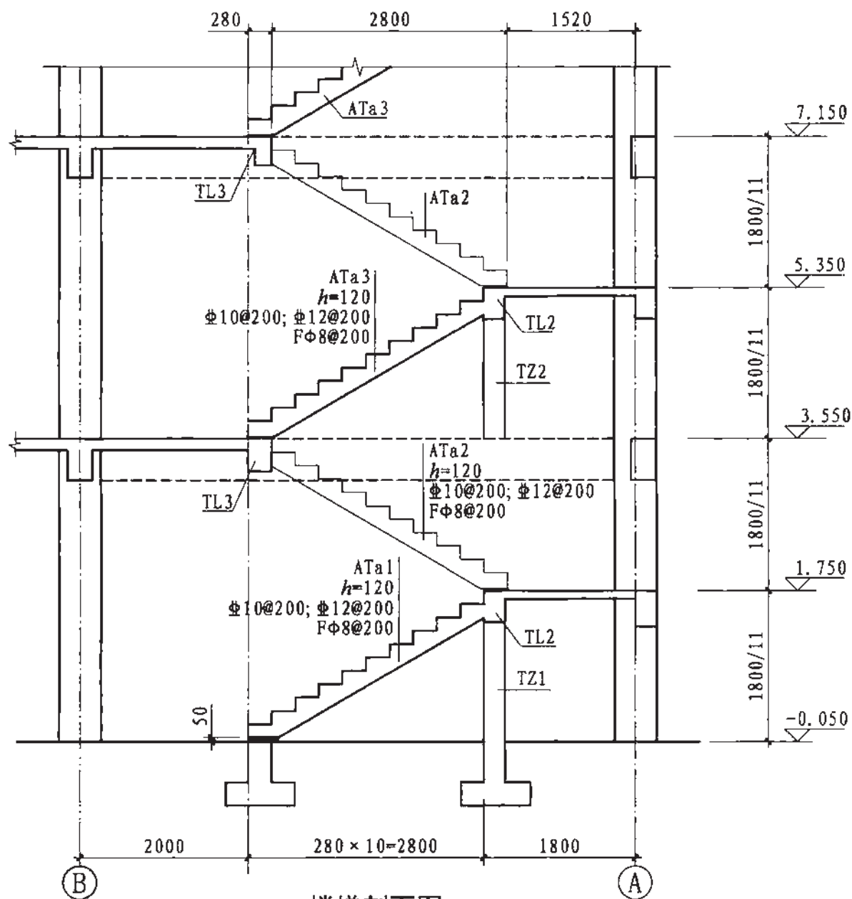
楼梯剖面图 局部示意
