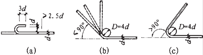
钢筋弯钩构造
