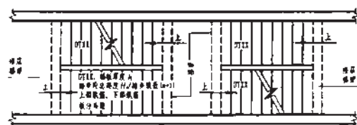
图5 剪刀楼梯
