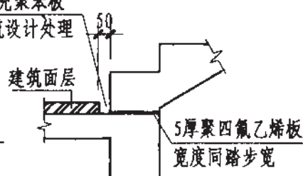
(2) 设聚四氟乙烯垫板 (梯段浇筑时应在垫板上铺塑料薄膜)
