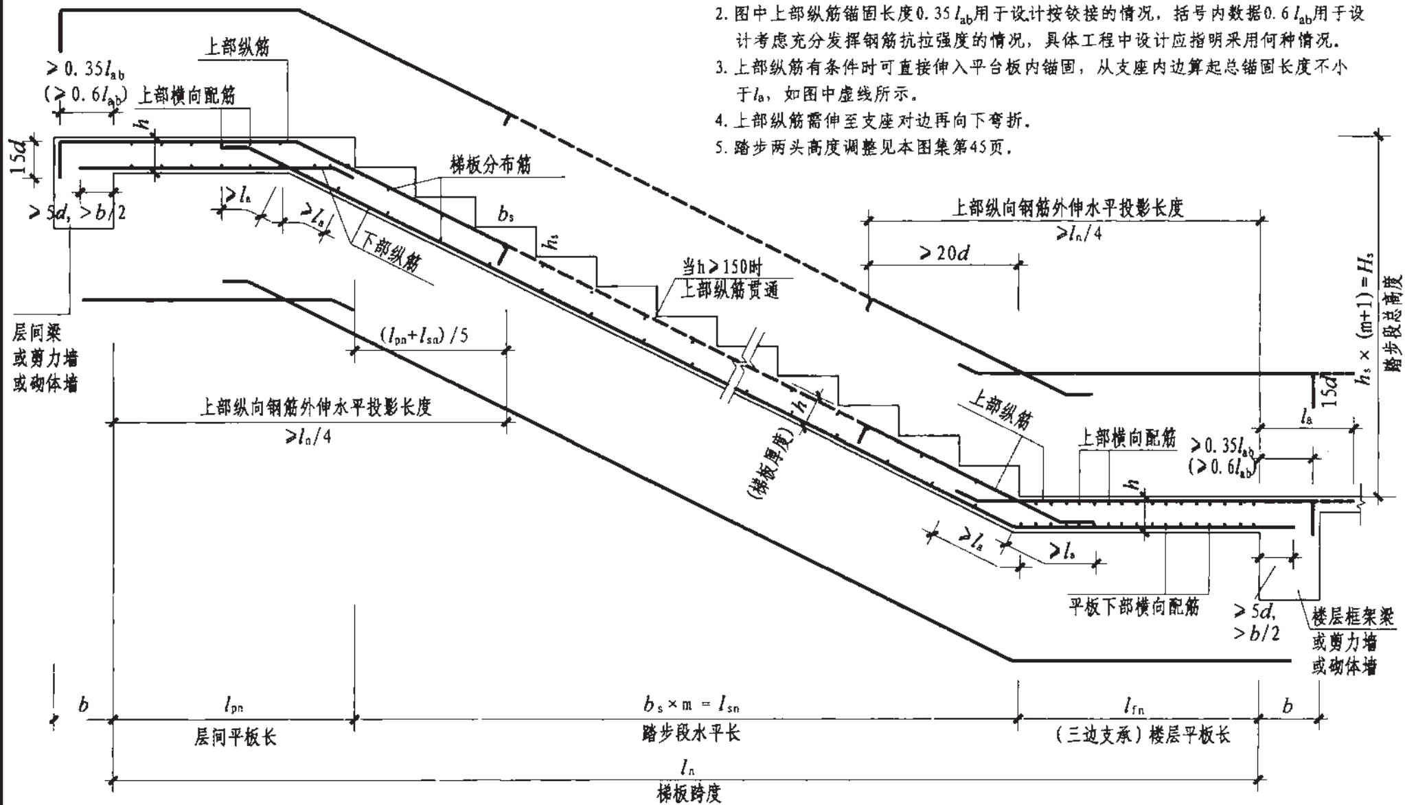
GT楼梯板配筋构造 (A-A) (楼层平板为三边支承，层间平板为单边支承)
