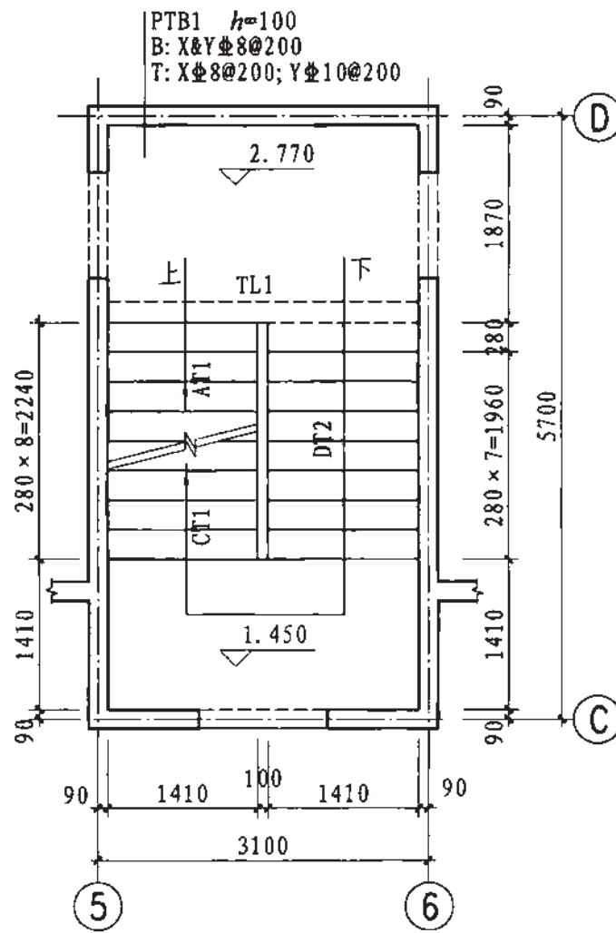
▽ 1.450 ~ 2.770 楼梯平面图
