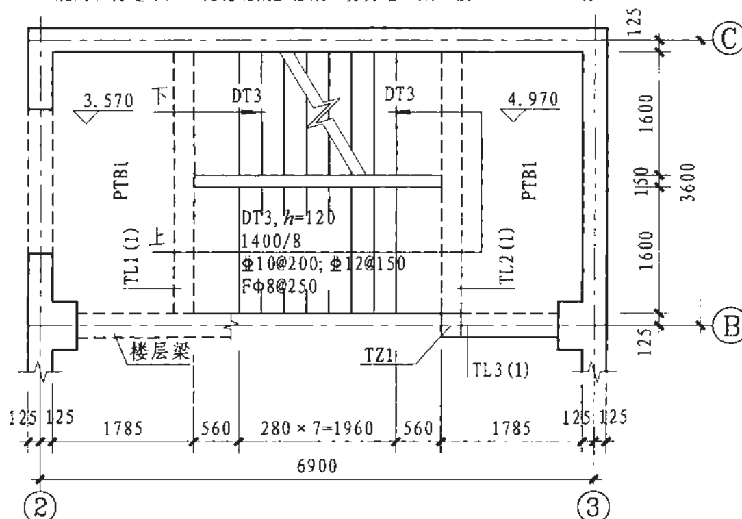
图2 设计示例 \nabla 3.570— \nabla 4.970楼梯平面图
