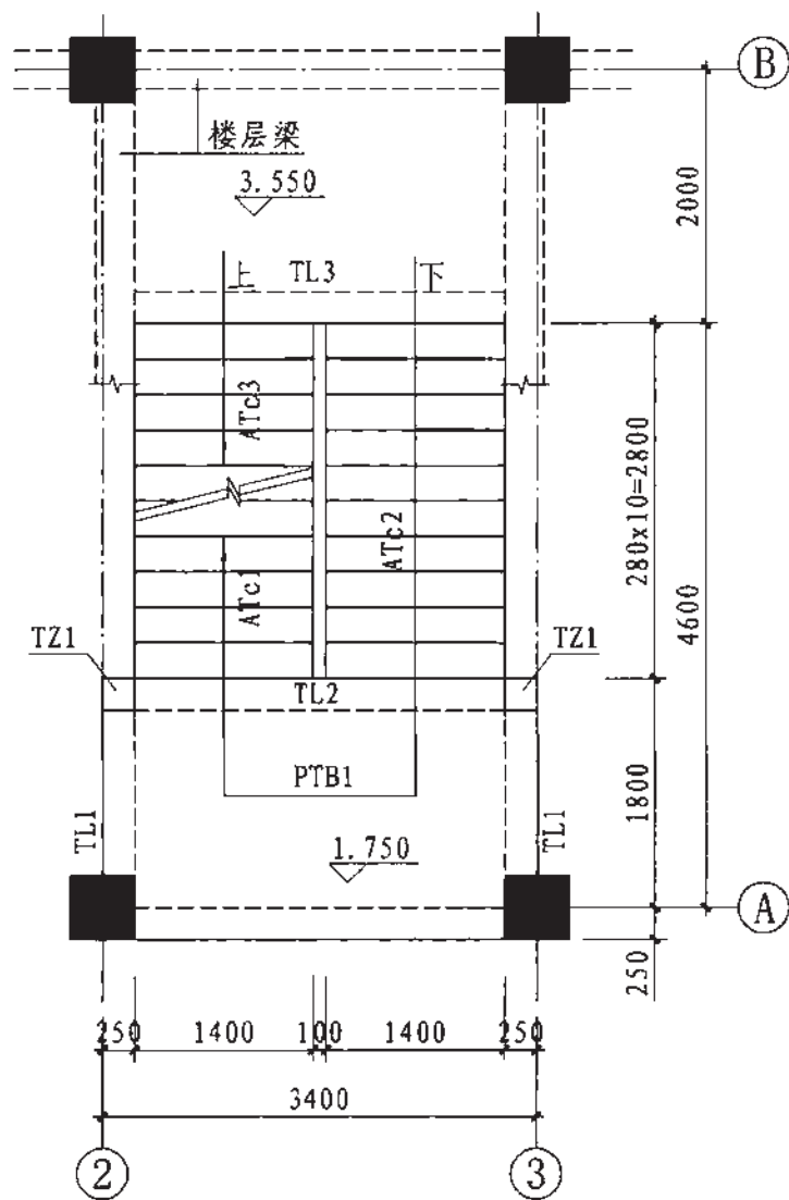
二层平面图
