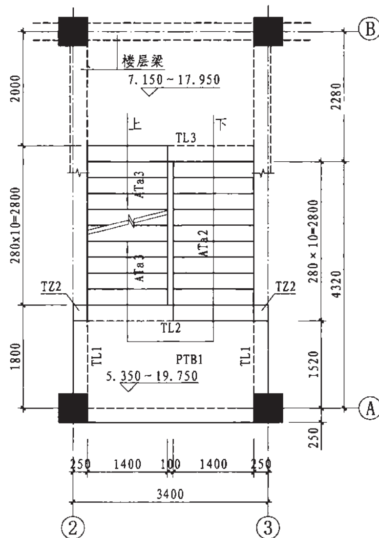
标准层平面图
