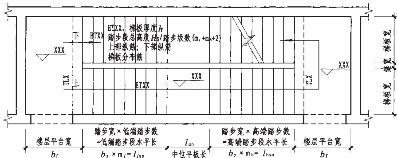
标高XXX—标高XXX楼梯平面图
