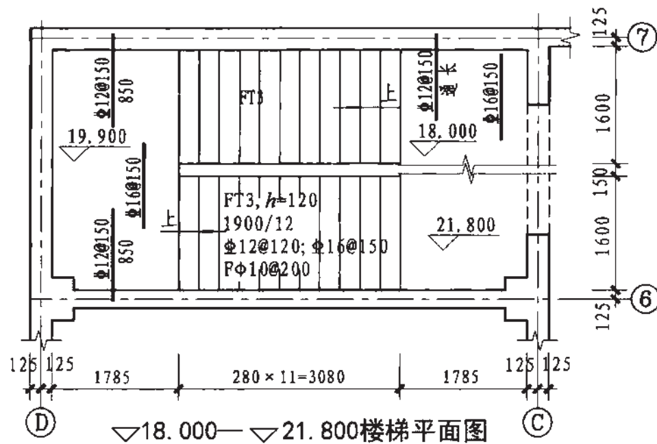
图2 设计示例
