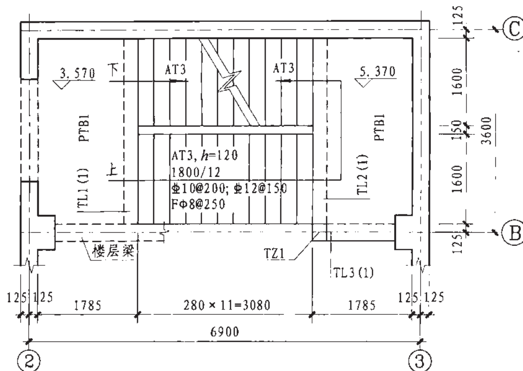
图2. 设计示例 \nabla 3.570— \nabla 5.370楼梯平面图
