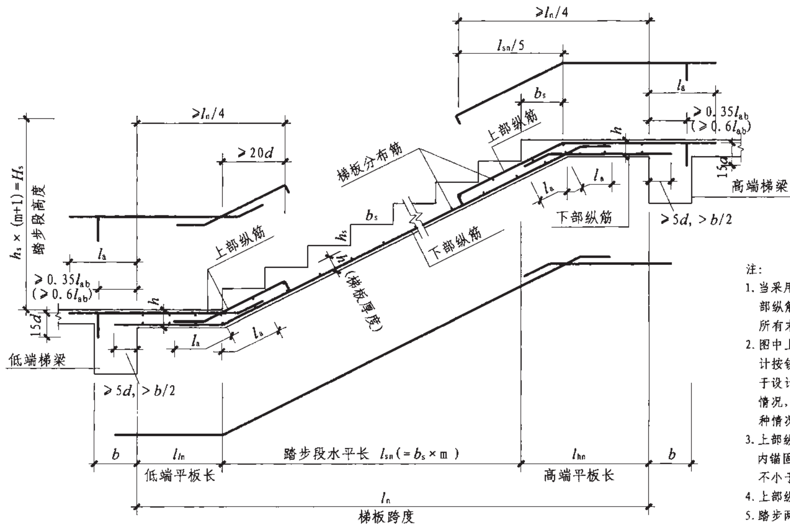
DT型楼梯板配筋构造
