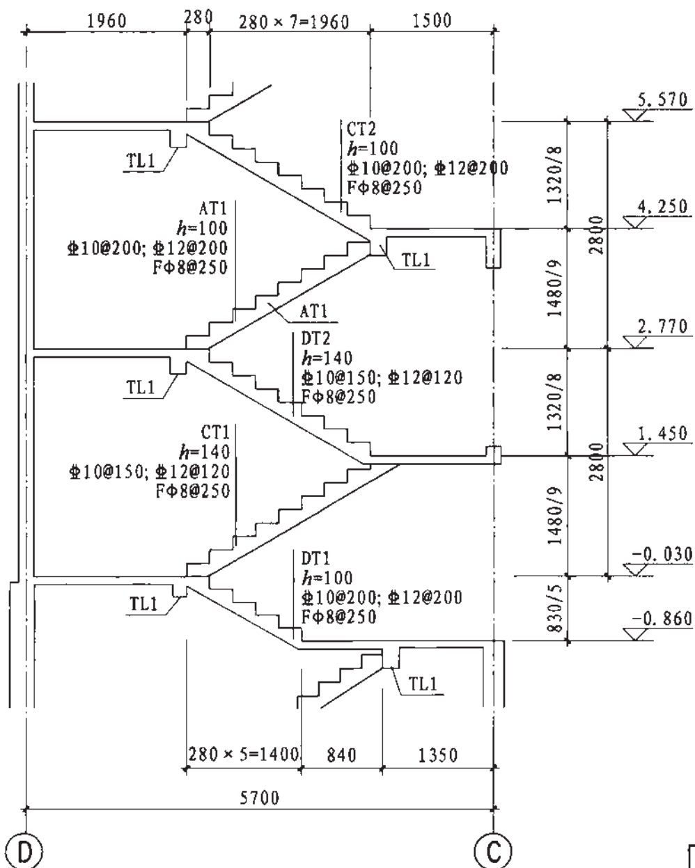
1-1剖面图
