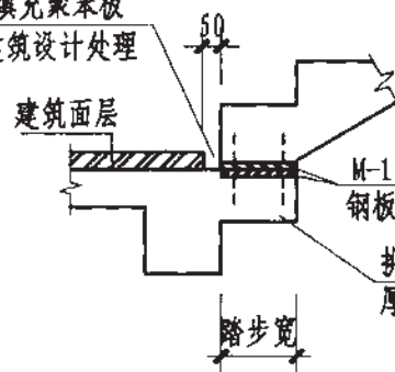
(1) 预埋钢板
