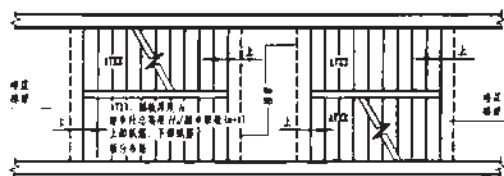
图5 剪刀楼梯
