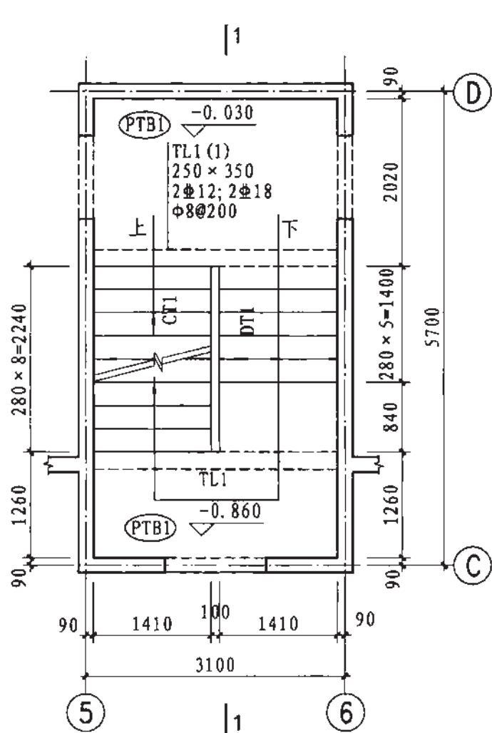
▽ -0.860 ~ -0.030 楼梯平面图
