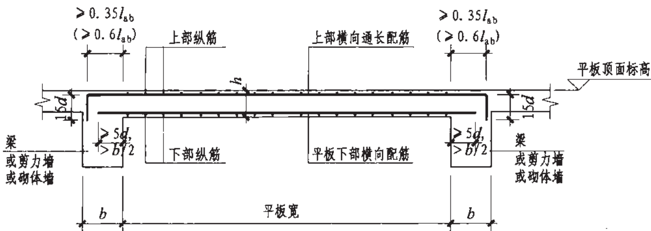
D-D剖面楼梯平板配筋构造
